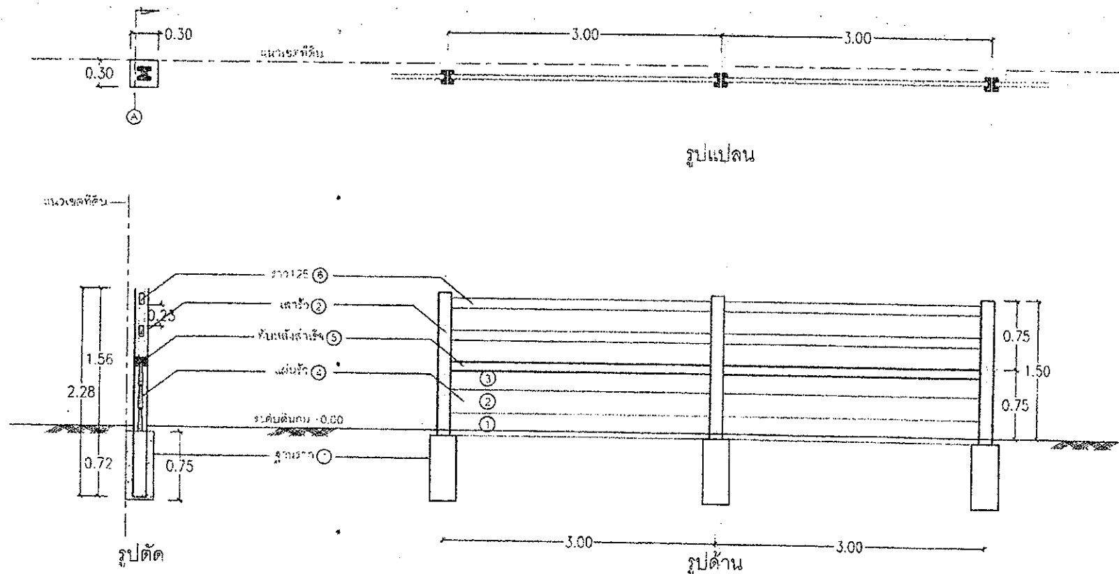
รูปตัด (SECTION A)
